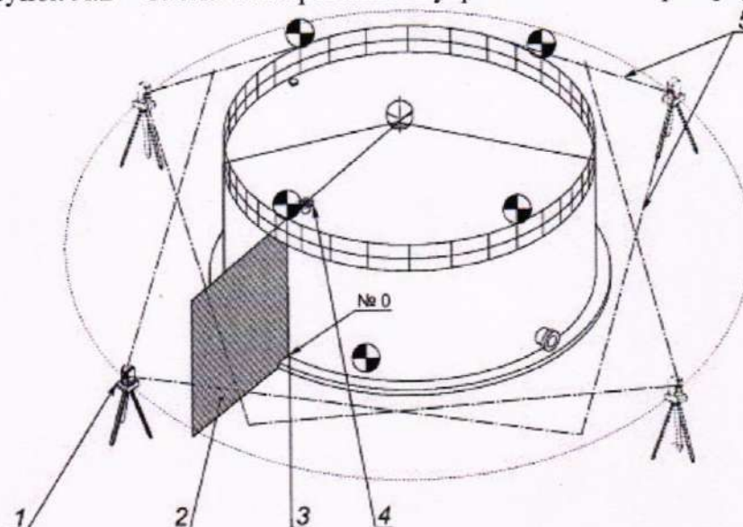
1 - станция сканирования; 2 - плоскость A; 3 - сферическая марка, установленная на ограждении кровли; 4 - точка измерения базовой высоты; 5 - сектор сканирования; сферическая марка
