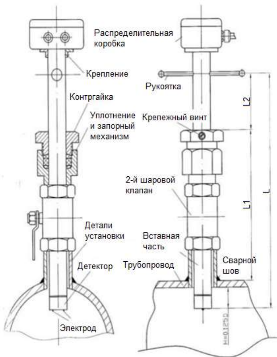
Рисунок 1. Конструкция ПП с шаровым краном
