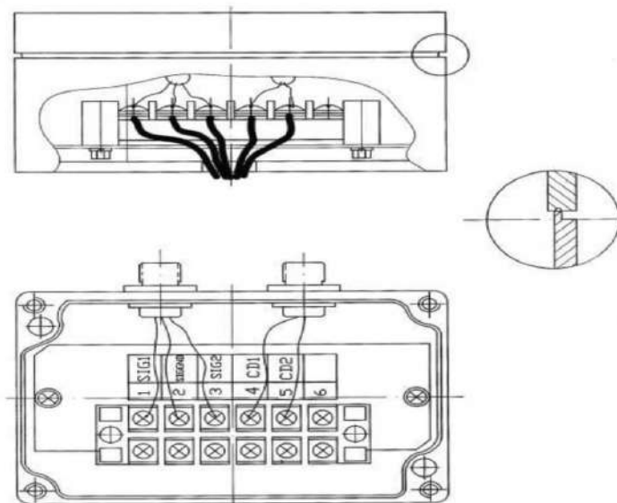
Рисунок 11. Схема подключения распределительной коробки
