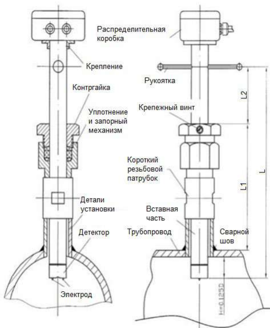
Рисунок 2. Конструкция ПП без шарового крана
