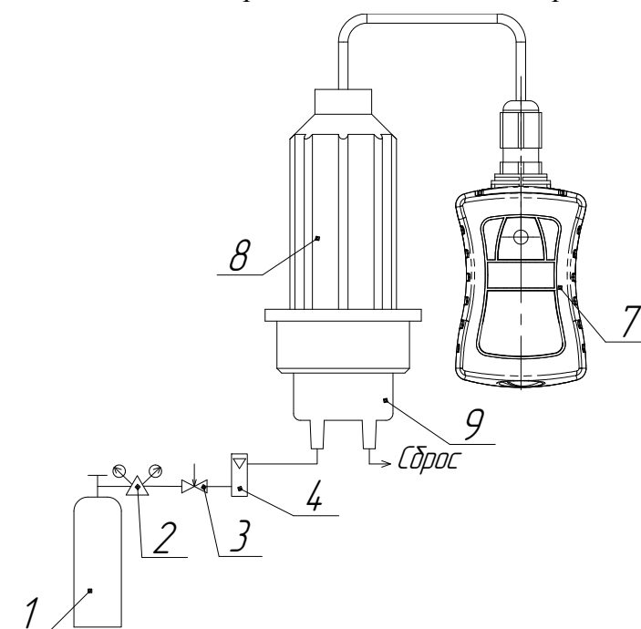
а) газоанализаторы АНКАТ-7631Микро-СО, АНКАТ-7631Микро-О 2 , АНКАТ-7631Микро-НН 3
