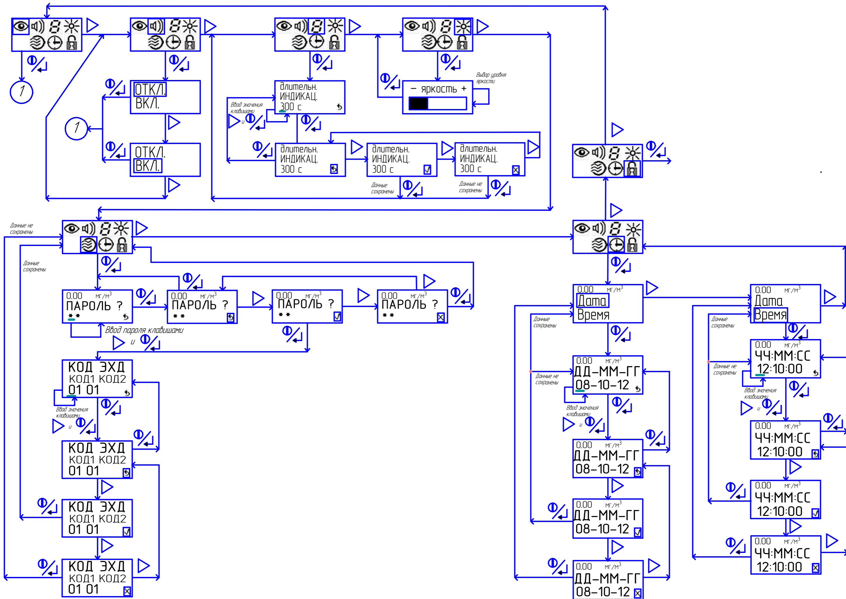
Рисунок Г.4 - Схема режимов работы. Режим настройки газоанализаторов
