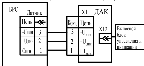
Схема электрическая подключений газоанализаторов к БРС (ИБЯЛ.411111.036-01, -02)
