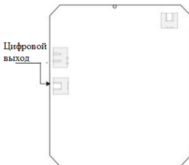
Рисунок 8. Подключение цифрового выхода ВП MT150НС (клеммы располагаются на задней стороне платы главного экрана)
