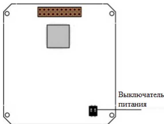
Рисунок 5. Выключатель питания вторичного преобразователя MT150НС, находится под платой главного экрана
