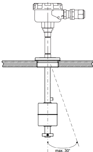
Рисунок 3. Монтаж сигнализатора на емкости
