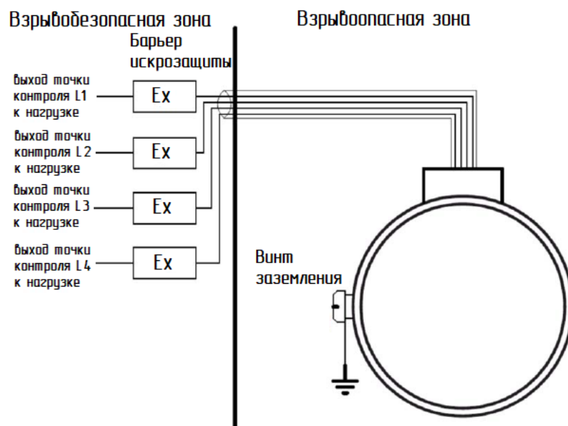
Рисунок Б.4 Пример подключения сигнализатора с видом взрывозащиты 0 Ex ia IIC T6 Ga X (4 точки контроля)
