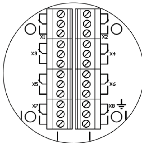
Рисунок Б.3 – Схема монтажная печатной платы сигнализатора РИЗУР-М-В на 1 ... 8 точек контроля
