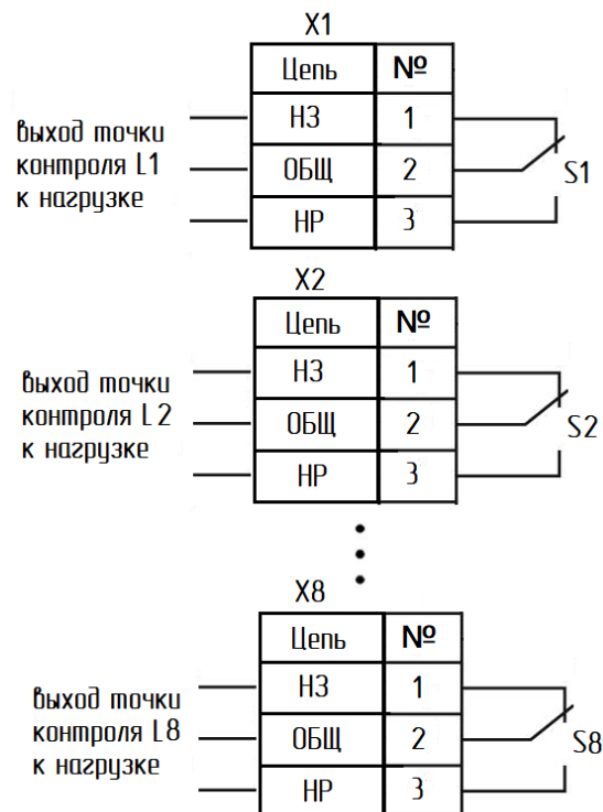
Рисунок Б.1 – Схема электрическая принципиальная – подключения сигнализатора РИЗУР-М-В на 1 ... 8 точек контроля (состояние контактов указано при отсутствии жидкости в точках контроля).
