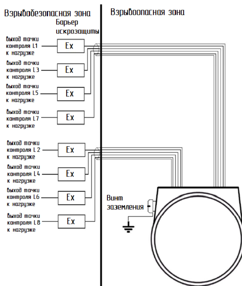
Рисунок Б.5 Пример подключения сигнализатора с видом взрывозащиты 0 Ex ia IIC T6 Ga X.
