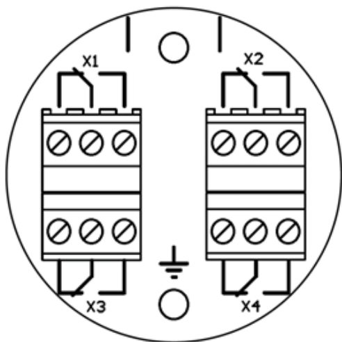
Рисунок Б.2 – Схема монтажная печатной платы сигнализатора РИЗУР-М-В на 1 ... 4 точки контроля.
