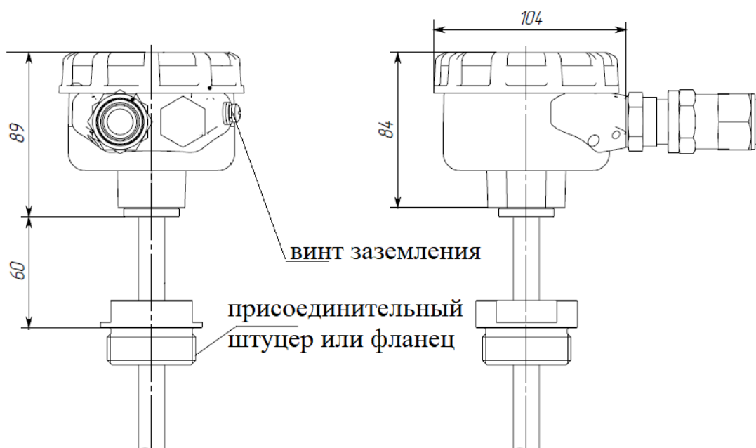
Рисунок А.2 Габаритные размеры сигнализатора с корпусом А100, Н100 для 1 ... 8 точек контроля
