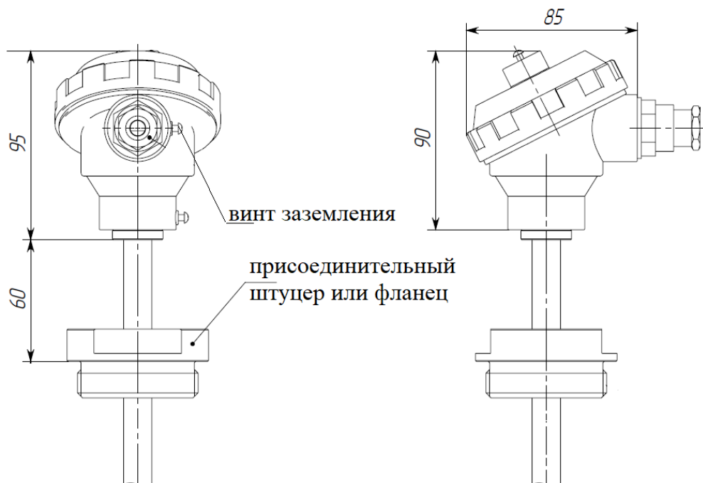
Рисунок А.1 Габаритные размеры сигнализатора с корпусом А80 для 1 ... 4 точек контроля.
