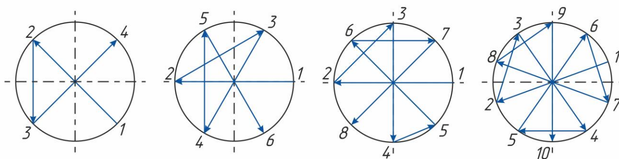
Рисунок 4. Последовательность затяжки фланцевых соединений
