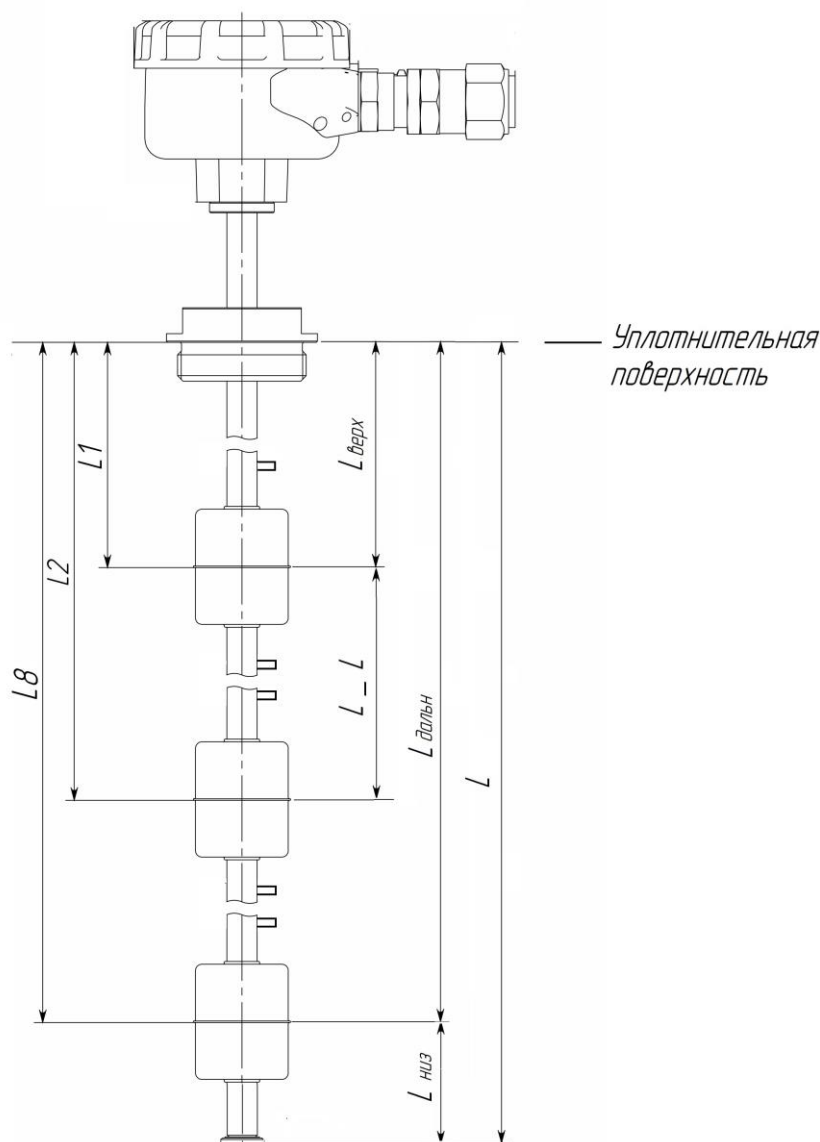
Рисунок 2. Технологические размеры, нумерация и расположение точек контроля.
