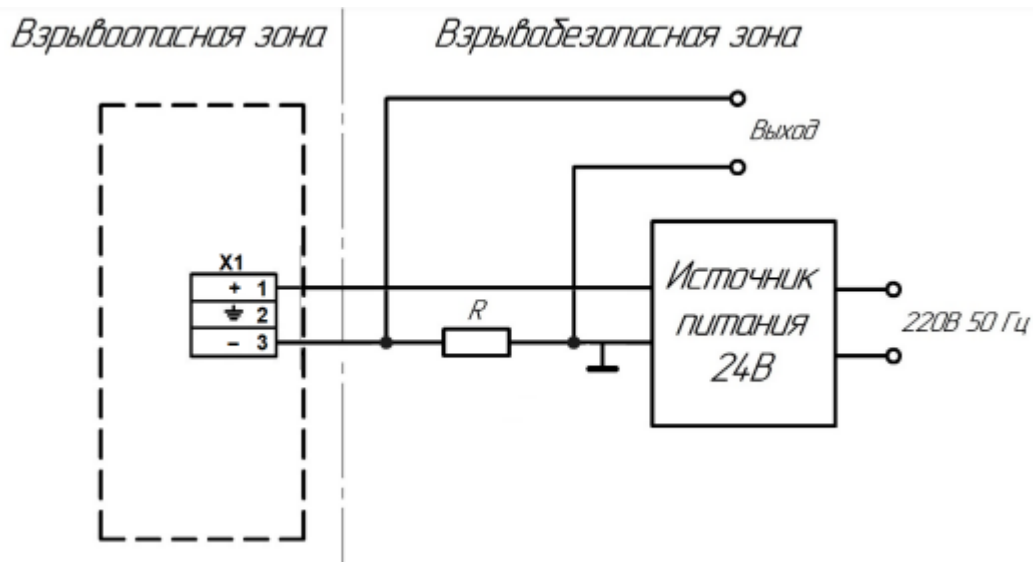
Рисунок А.3 Пример подключения сигнализатора РИЗУР-М-П «токовая петля» (для выходного сигнала 4/20мА: отсутствие жидкости 4 мА, наличие - 20 мА; для выходного сигнала 7/14мА: отсутствие жидкости 7 мА, наличие - 14 мА; для выходного сигнала 8/16мА: отсутствие жидкости 8 мА, наличие - 16 мА)
