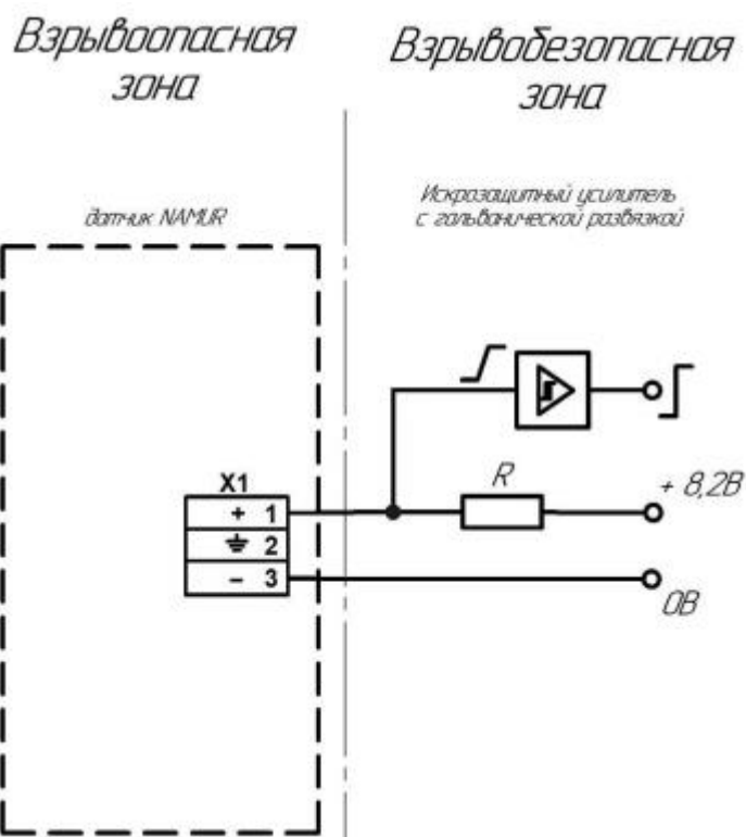
Рисунок А.4 Пример подключения сигнализатора РИЗУР-М-П «NAMUR» (для выходного сигнала Namur: отсутствие жидкости 0.2..1.2 мА, наличие - 2.1..6.5 мА)
