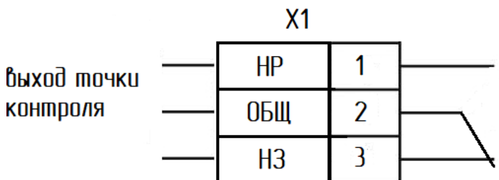
Рисунок А.1 – Схема электрическая принципиальная – подключения сигнализатора РИЗУР-М-П «сухой контакт» (состояние контактов указано при отсутствии жидкости в точке контроля).
