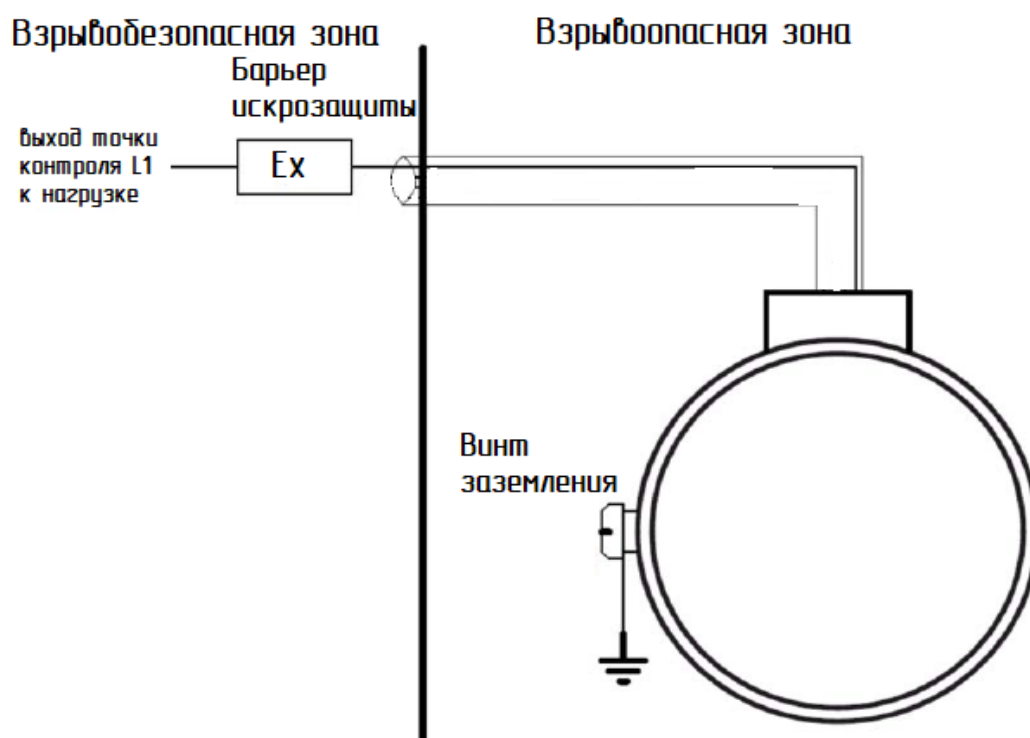
Рисунок А.2 Пример подключения сигнализатора РИЗУР-М-П с видом взрывозащиты 0 Ex ia IIC T6 Ga X
