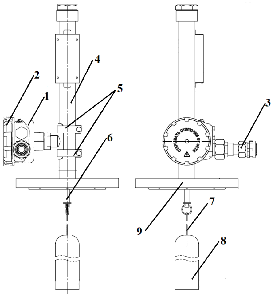
Рисунок 1. Внешний вид сигнализатора
