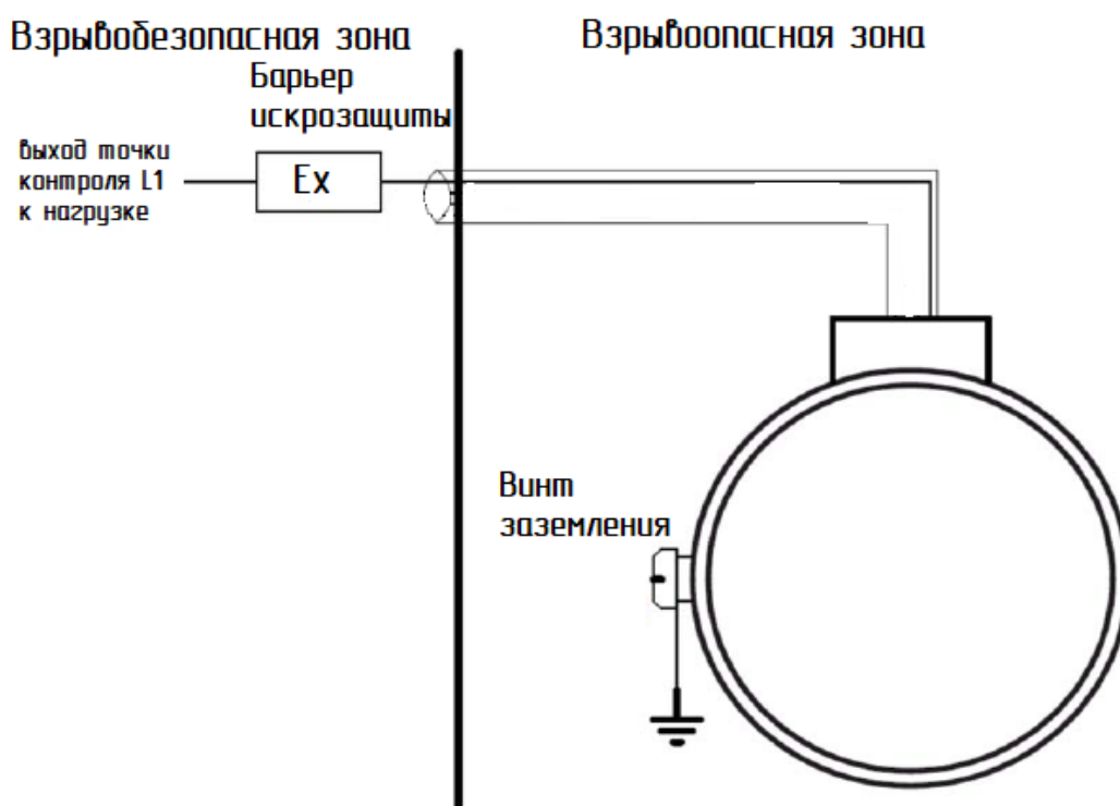
Рисунок А.2 Пример подключения сигнализатора РИЗУР-М-Б с видом взрывозащиты 0 Ex ia IIC T6 Ga X
