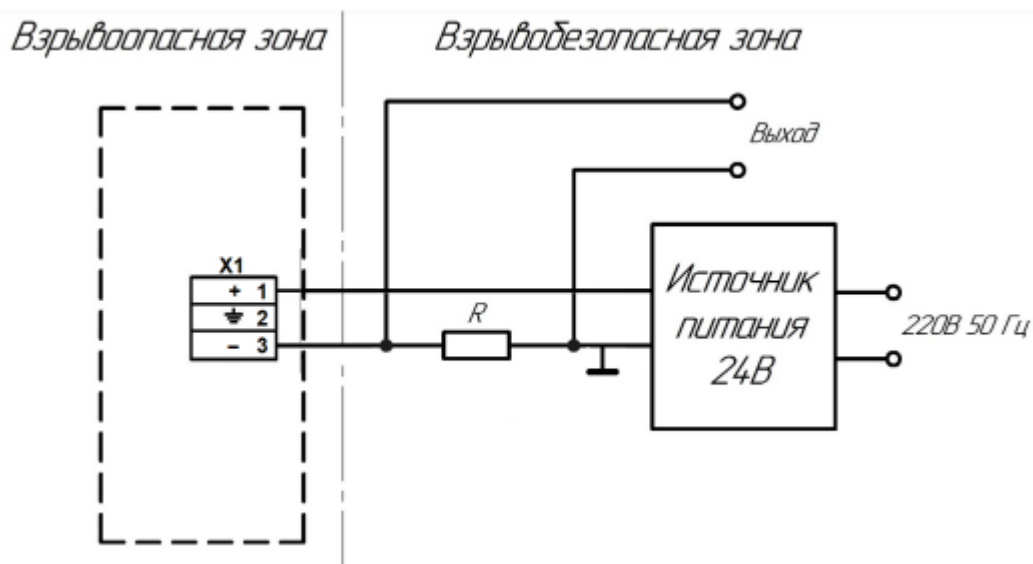
Рисунок А.3 Пример подключения сигнализатора РИЗУР-М-Б «токовая петля» (для выходного сигнала 4/20мА: отсутствие жидкости 4 мА, наличие - 20 мА; для выходного сигнала 7/14мА: отсутствие жидкости 7 мА, наличие - 14 мА; для выходного сигнала 8/16мА: отсутствие жидкости 8 мА, наличие - 16 мА)
