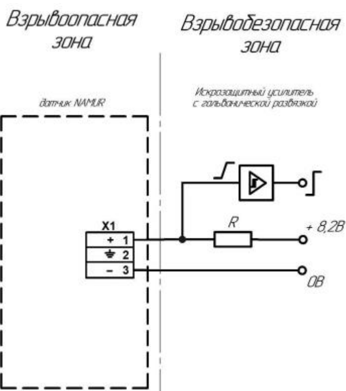
Рисунок А.4 Пример подключения сигнализатора РИЗУР-М-Б «NAMUR» (для выходного сигнала Namur: отсутствие жидкости 0.2..1.2 мА, наличие - 2.1..6.5 мА)
