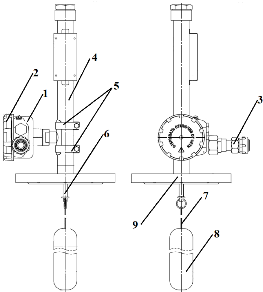
Рисунок 1. Внешний вид сигнализатора
