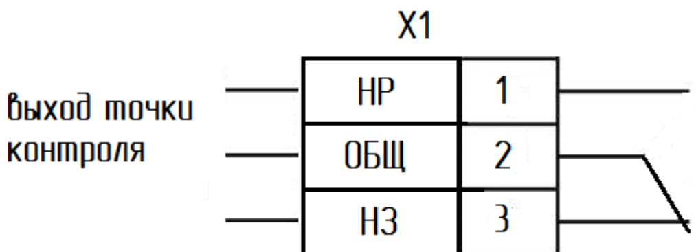
Рисунок А.1 – Схема электрическая принципиальная – подключения сигнализатора РИЗУР-М-Б «сухой контакт» (состояние контактов указано при отсутствии жидкости в точке контроля).
