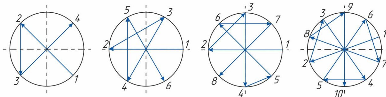
Рисунок 3. Последовательность затяжки фланцевых соединений
